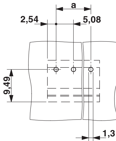
Bohrplan/Lötpadgeometrie
