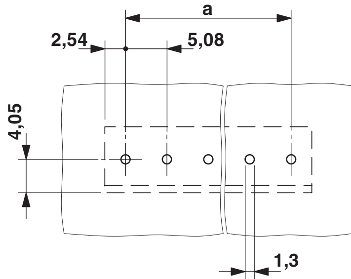
Bohrplan/Lötpadgeometrie
