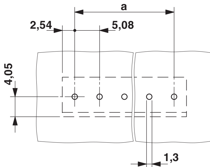
Bohrplan/Lötpadgeometrie
