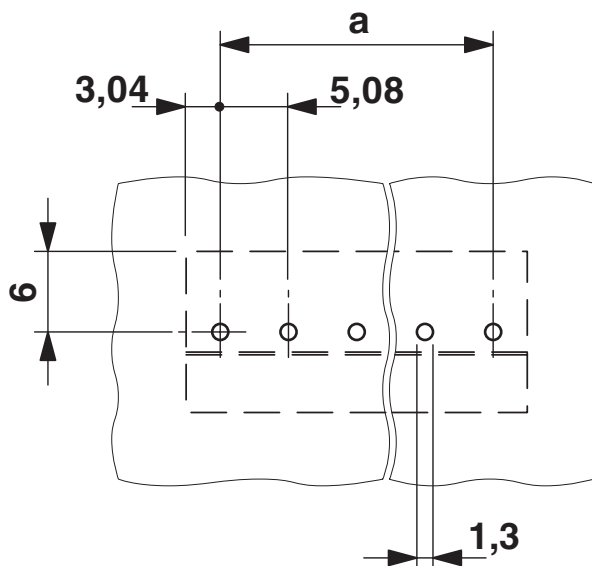
Bohrplan/Lötpadgeometrie
