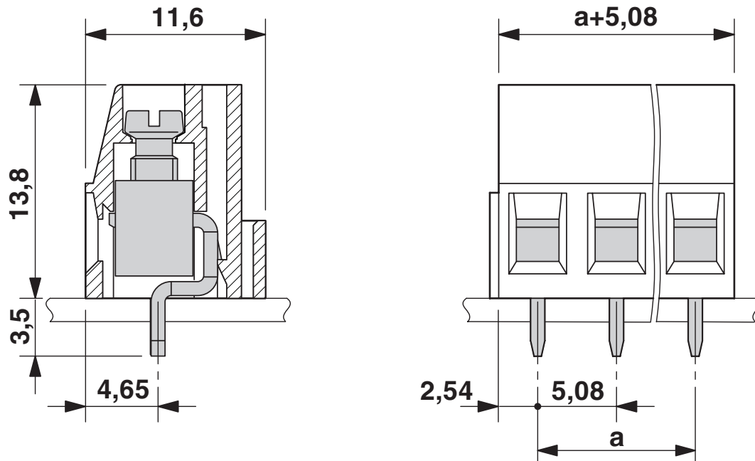
Maßzeichnung
