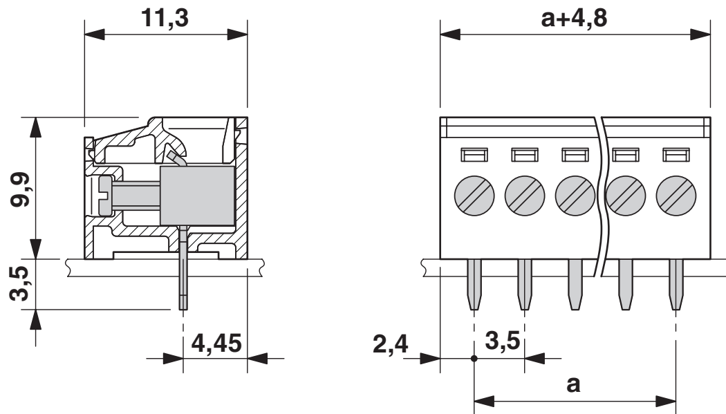
Maßzeichnung
