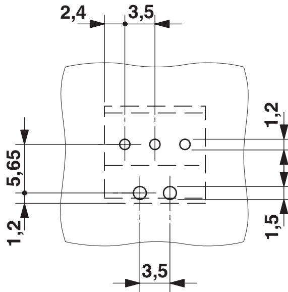
Bohrplan/Lötpadgeometrie
