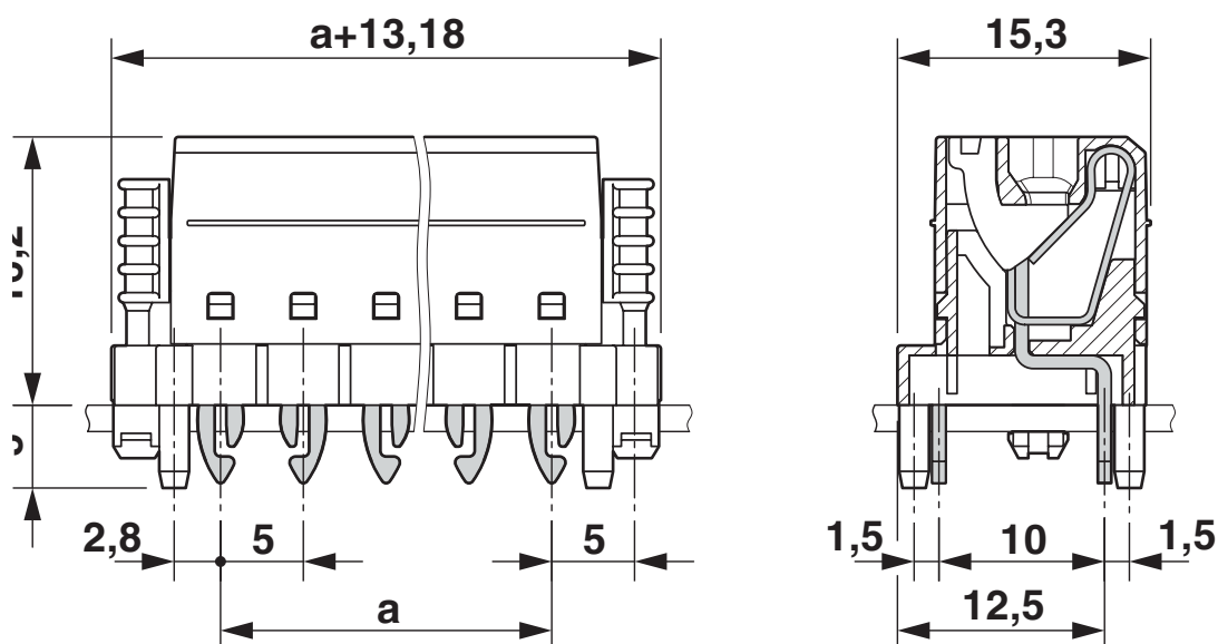
Maßzeichnung
