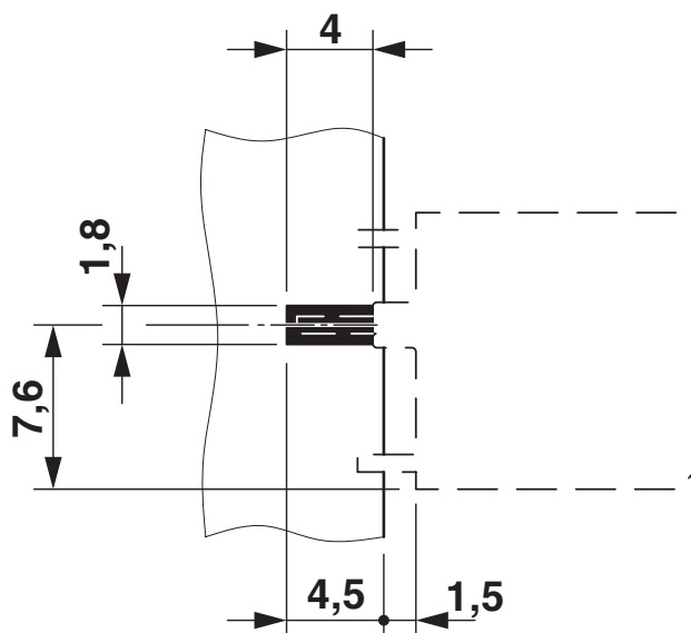
Bohrplan/Lötpadgeometrie
