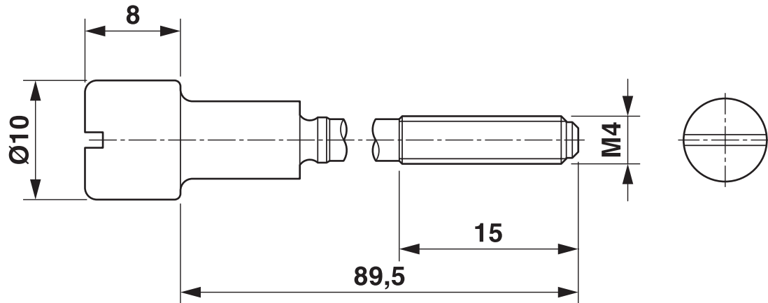
Maßzeichnung
