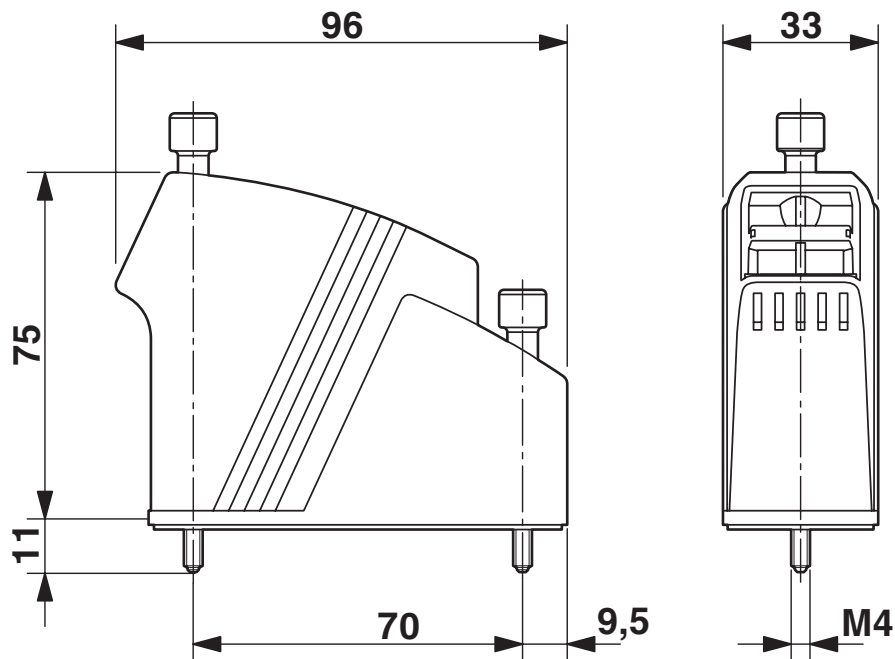
Maßzeichnung
