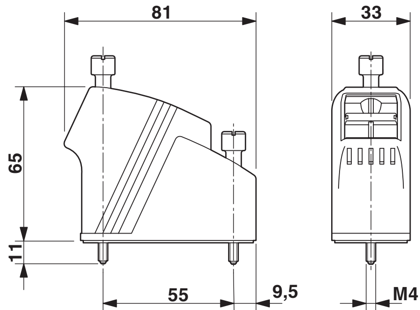
Maßzeichnung
