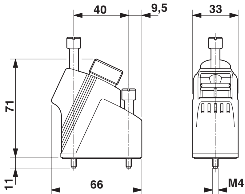
Maßzeichnung
