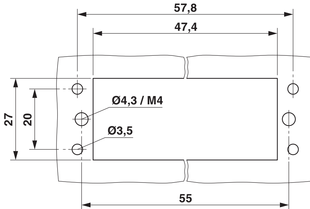
Maßzeichnung
