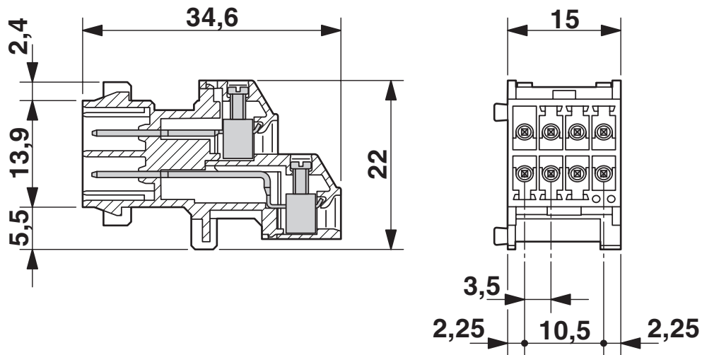
Maßzeichnung
