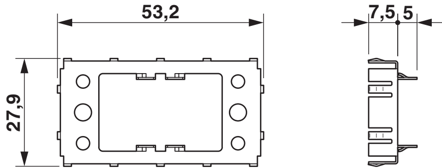
Maßzeichnung
