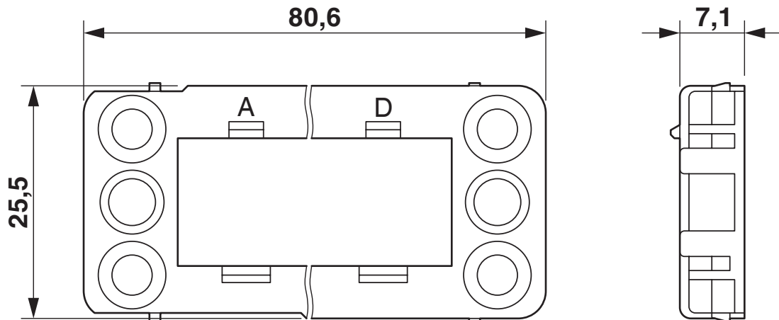
Maßzeichnung Anbaurahmen
