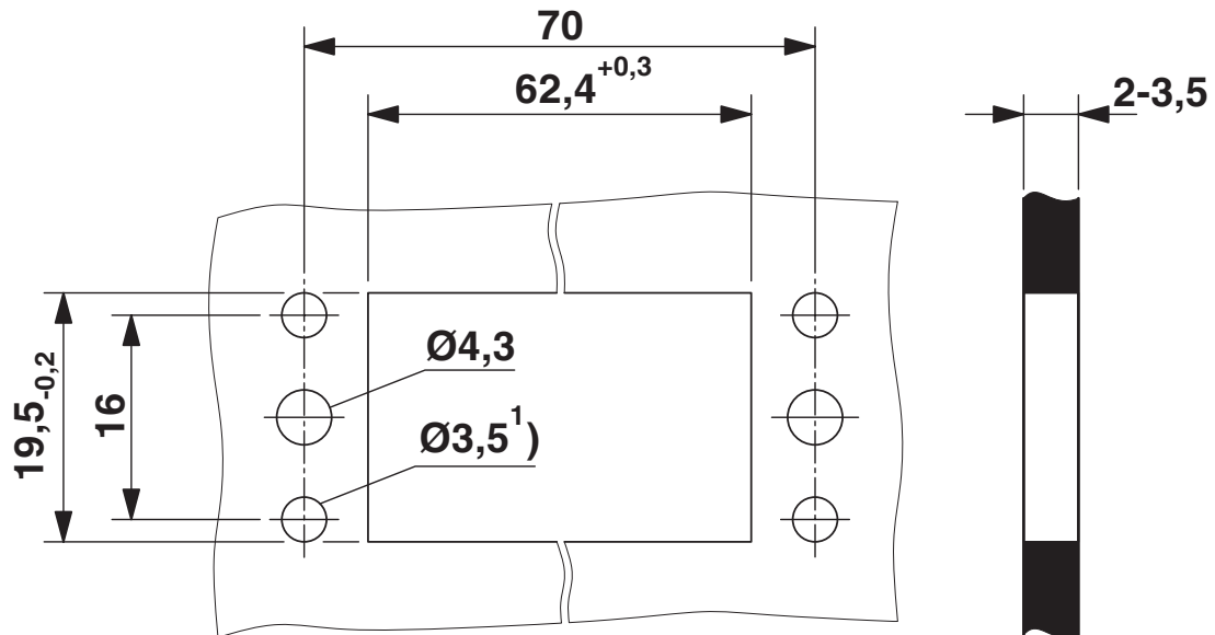
Maßzeichnung
