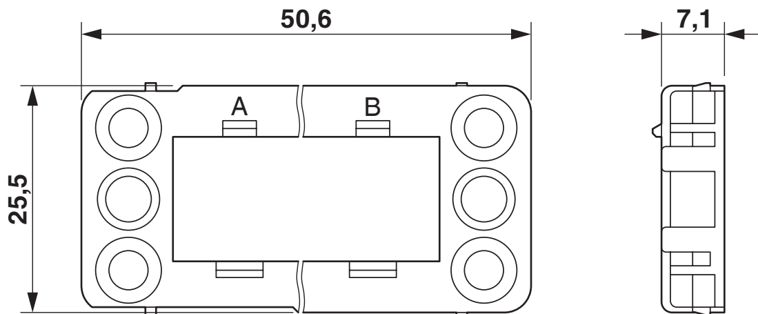
Maßzeichnung Anbaurahmen
