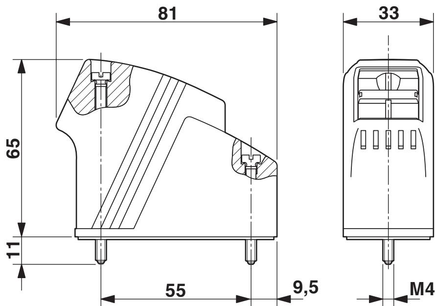
Maßzeichnung
