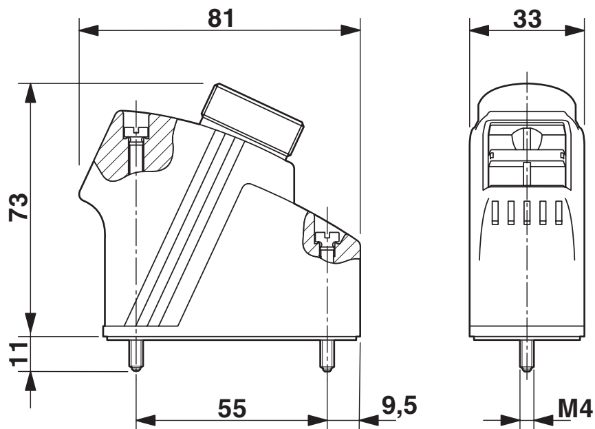
Maßzeichnung
