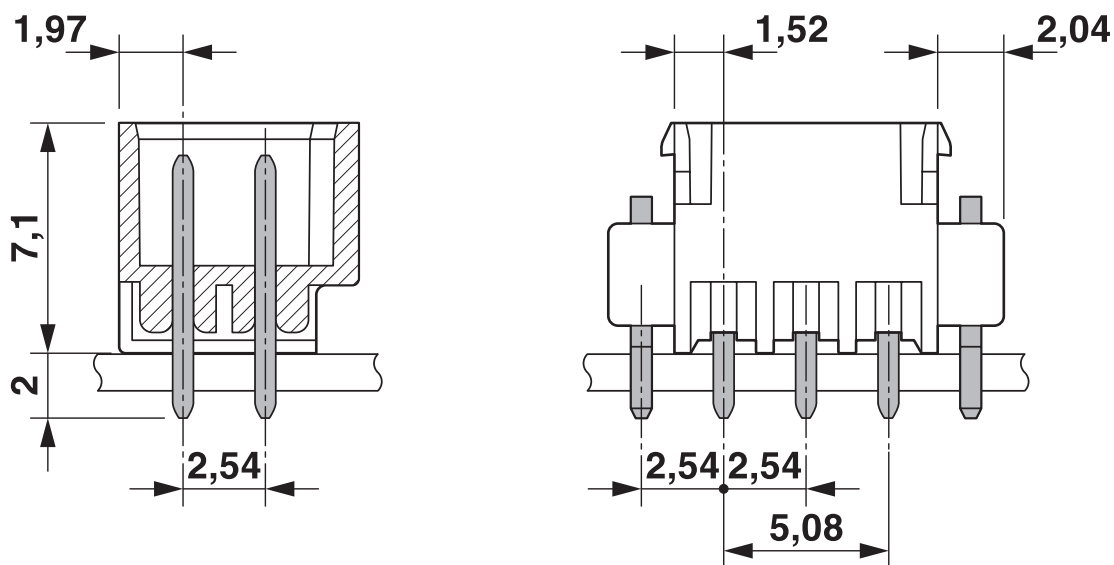
Maßzeichnung
