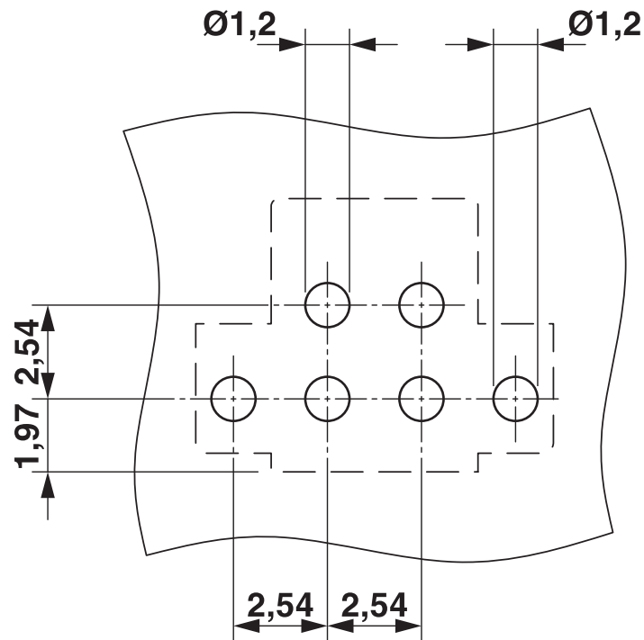
Bohrplan/Lötpadgeometrie
