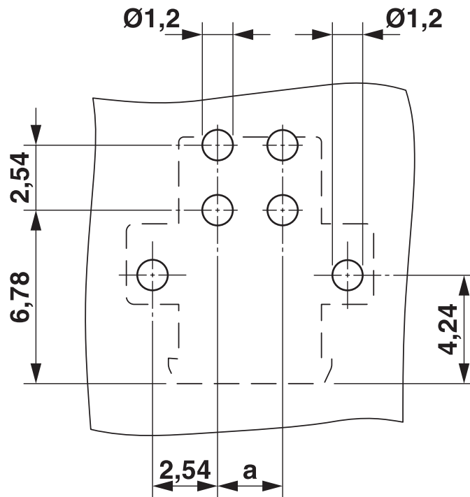
Bohrplan/Lötpadgeometrie
