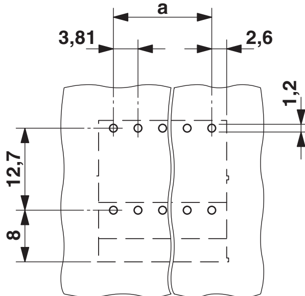
Bohrplan/Lötpadgeometrie
