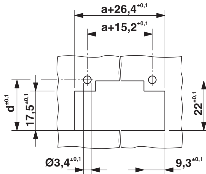
Maßzeichnung
