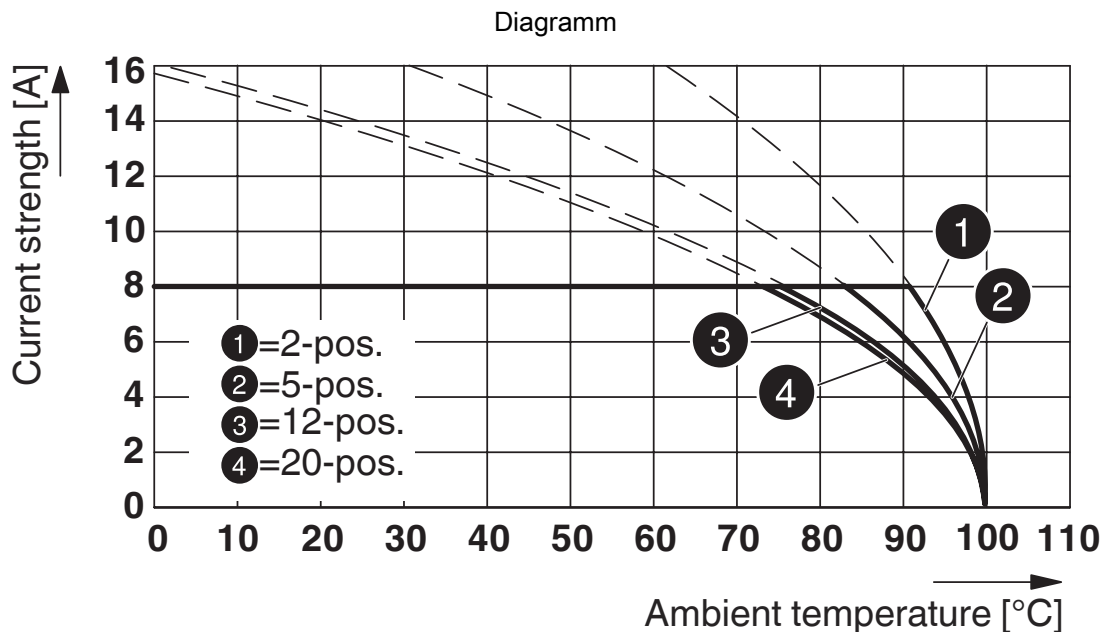
Typ: MC 1,5/...-ST-3,5 mit MCV 1,5/...-G-3,5
