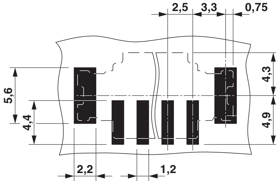
Bohrplan/Lötpadgeometrie
