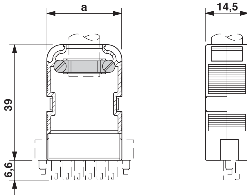
Maßzeichnung
