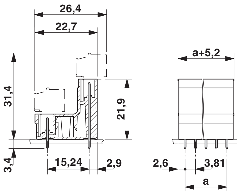
Maßzeichnung
