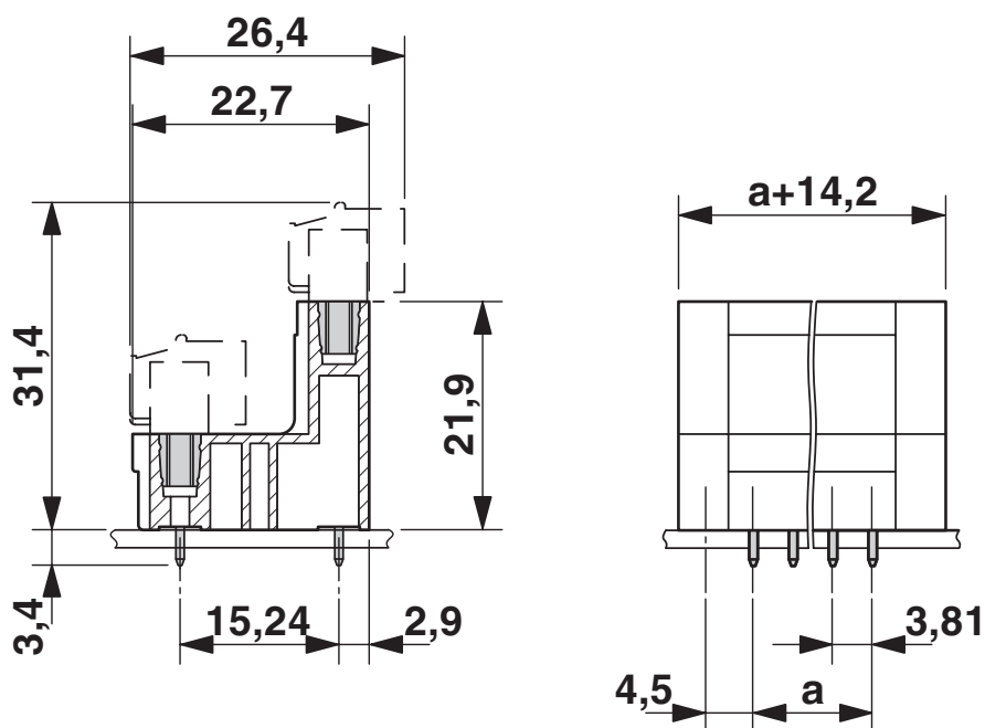
Maßzeichnung
