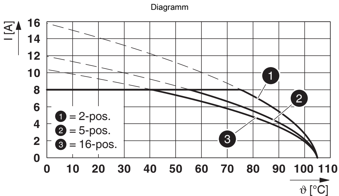
Typ: MCVR 1,5/...-STF-3,81 mit MCDV 1,5/...-GF-3,81
