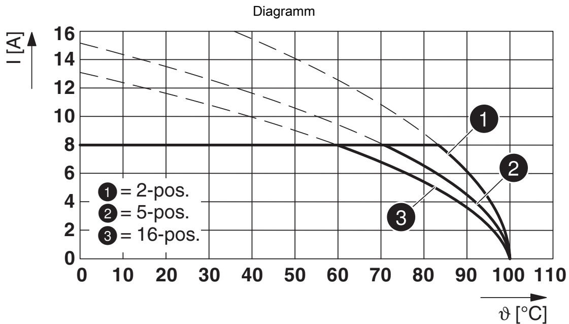
Typ: FMC 1,5/...-STF-3,81 mit MCDV 1,5/...-GF-3,81
