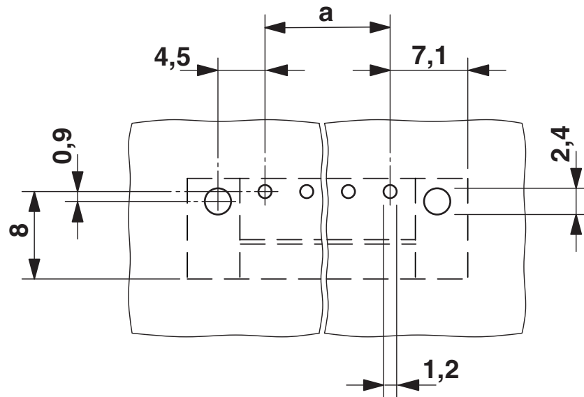
Bohrplan/Lötpadgeometrie
