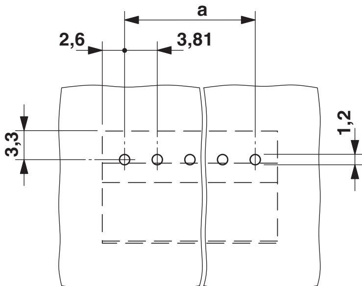
Bohrplan/Lötpadgeometrie
