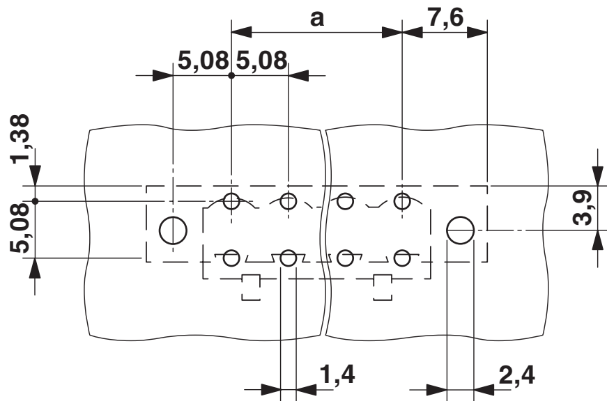
Bohrplan/Lötpadgeometrie
