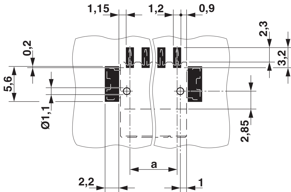
Bohrplan/Lötpadgeometrie
