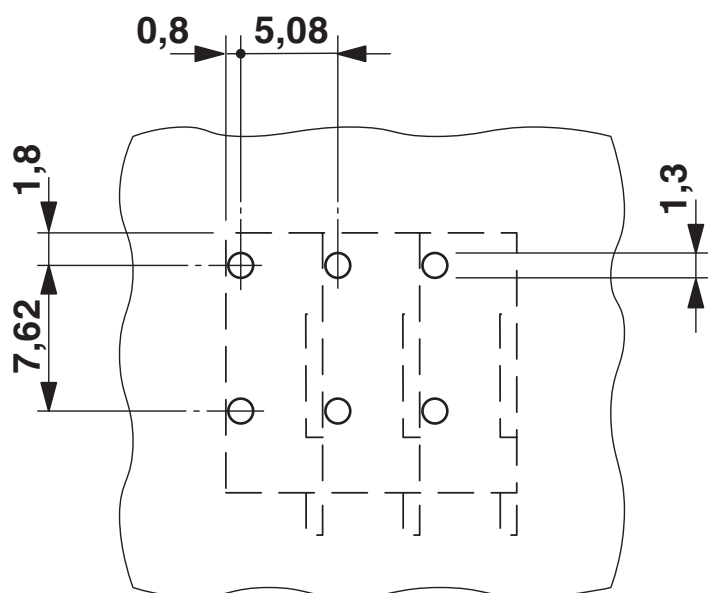
Bohrplan/Lötpadgeometrie
