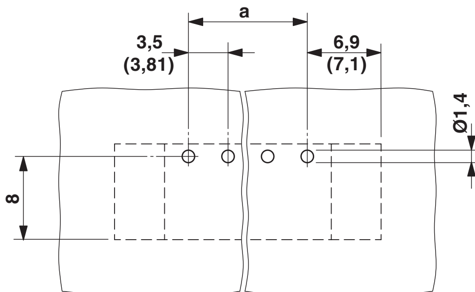
Bohrplan/Lötpadgeometrie
