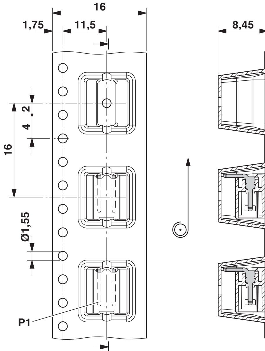
Maßzeichnung
