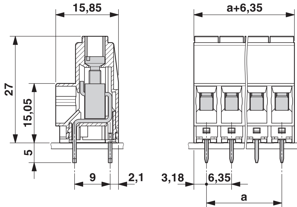
Maßzeichnung
