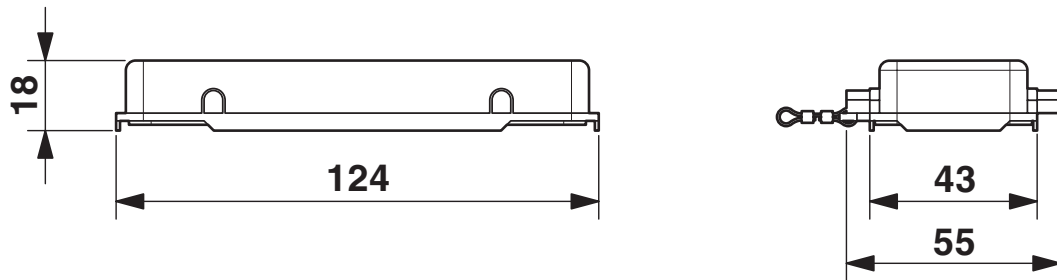
Maßzeichnung
