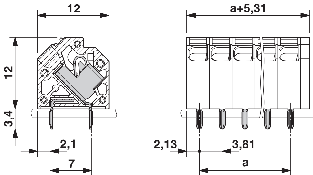
Maßzeichnung
