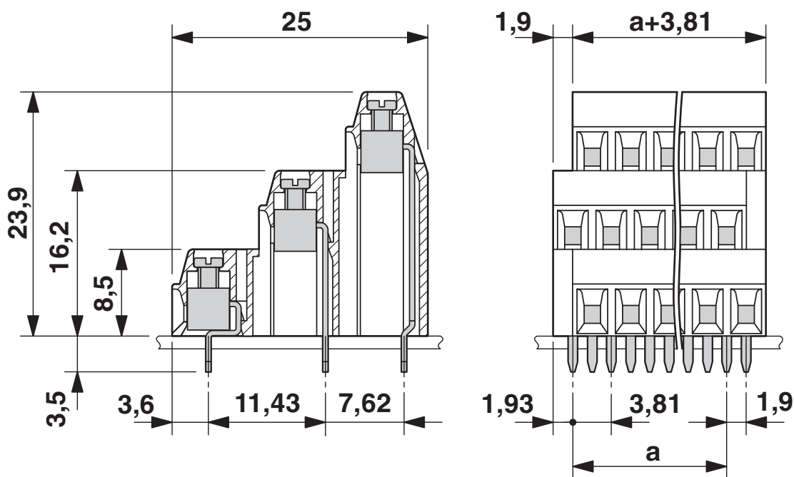
Maßzeichnung
