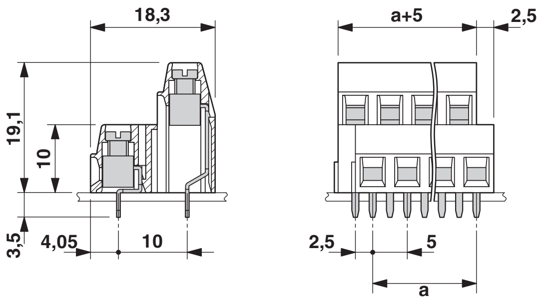
Maßzeichnung
