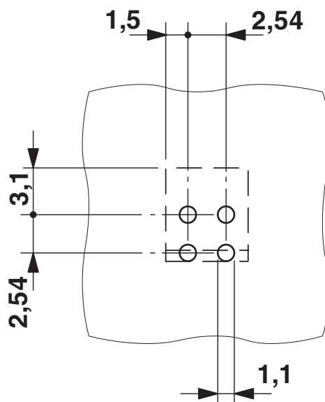
Bohrplan/Lötpadgeometrie
