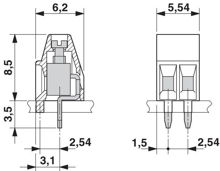
Maßzeichnung
