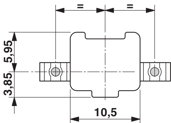
Maßzeichnung
