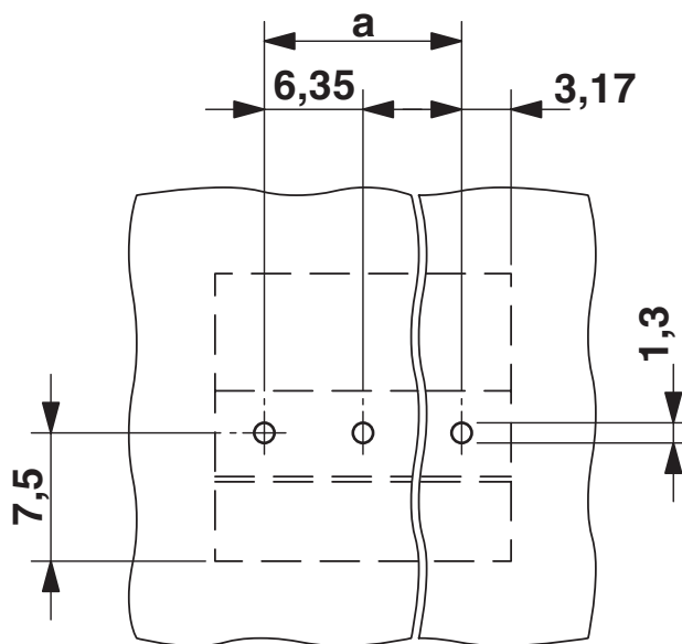
Bohrplan/Lötpadgeometrie
