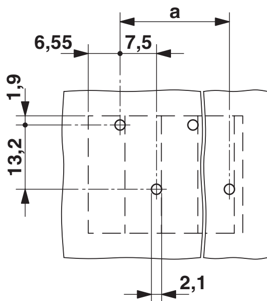
Bohrplan/Lötpadgeometrie
