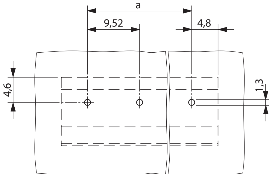
Bohrplan/Lötpadgeometrie
