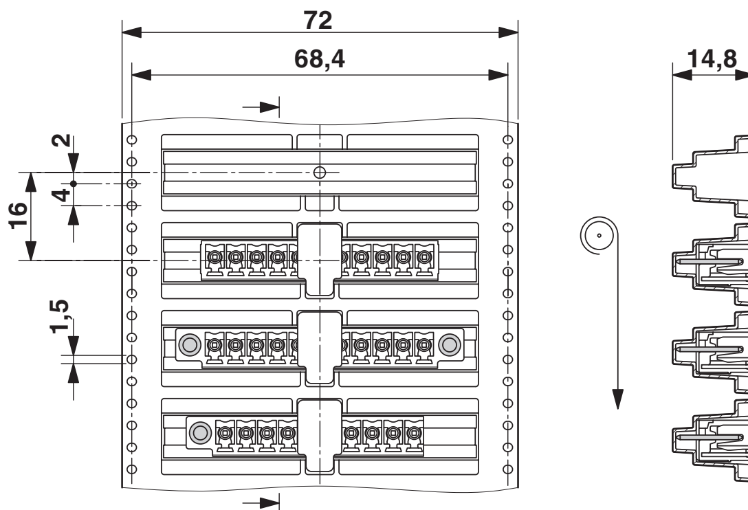
Maßzeichnung
