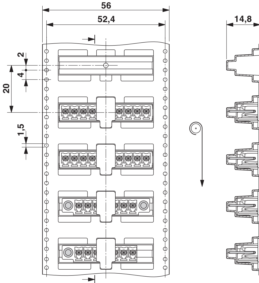
Maßzeichnung
