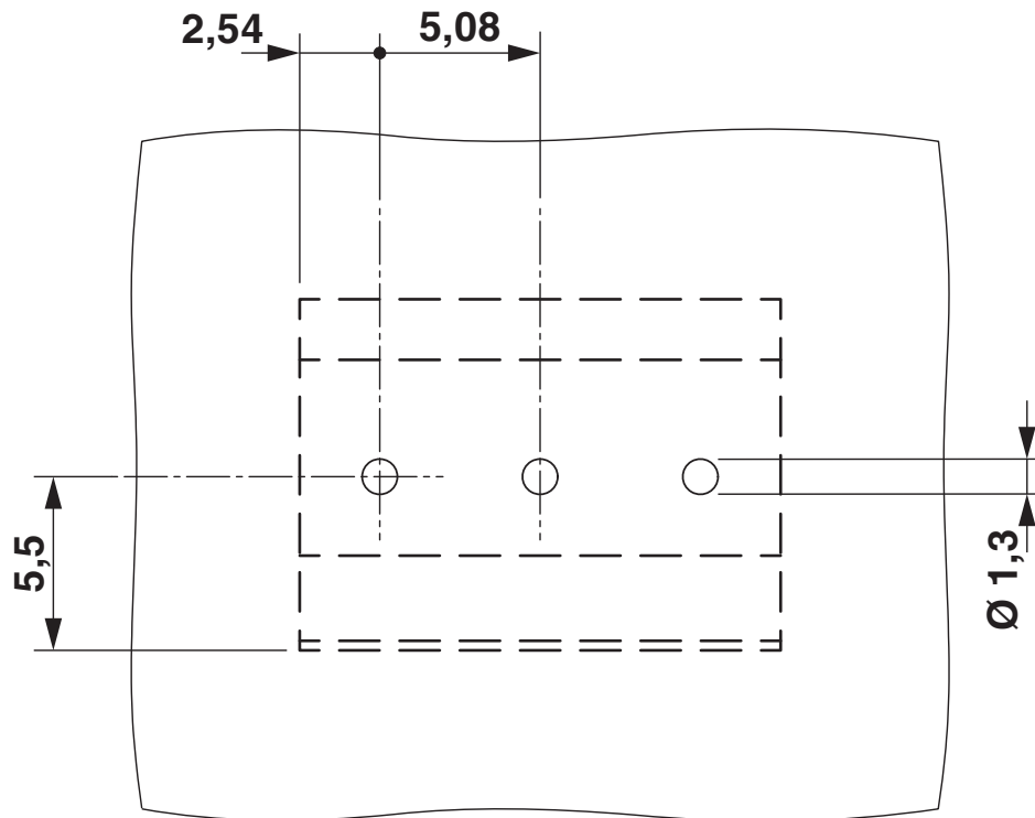
Bohrplan/Lötpadgeometrie
